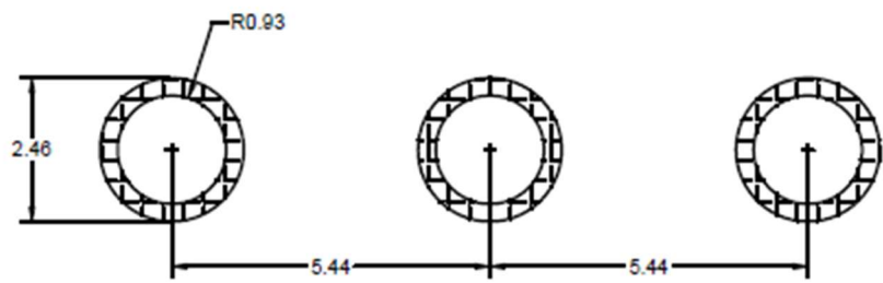
TO-247-3L
