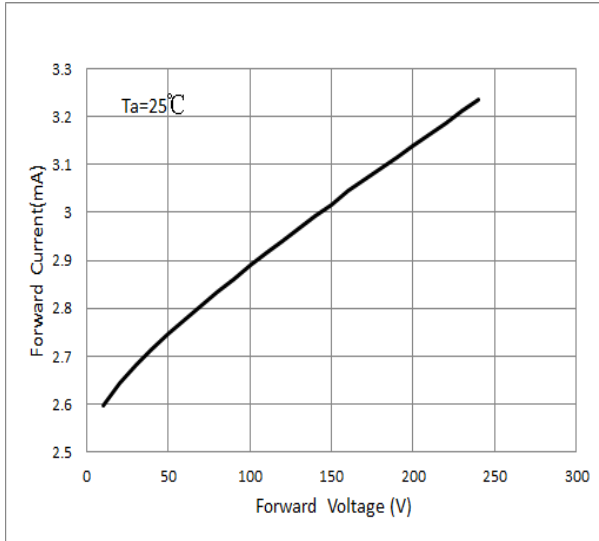
V_f ----- I_f
