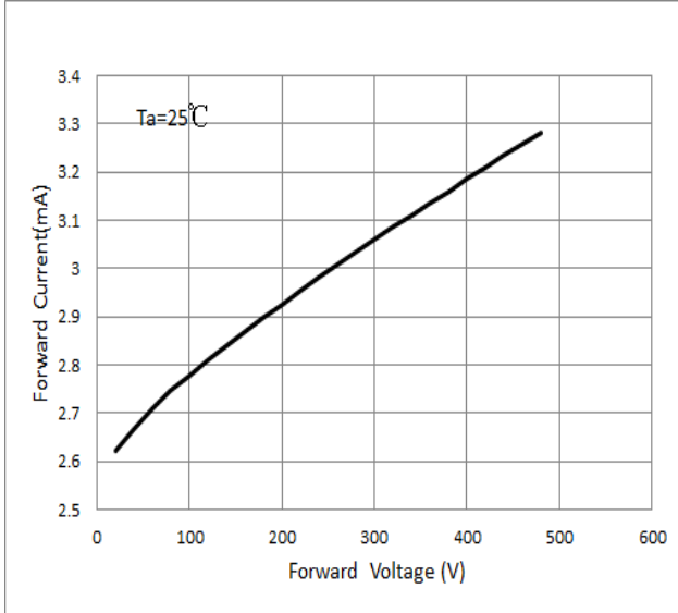
V_f ----- I_f
