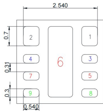
BOT VIEW
