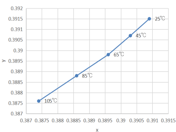
SOLDERING TEMP. VS. CIE X, Y SHIFT
